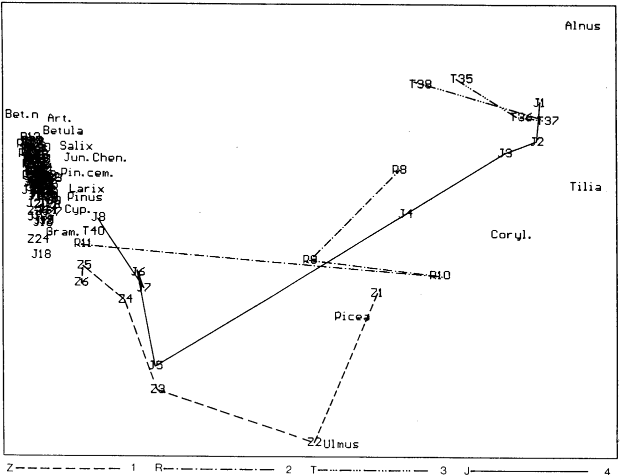
Fig. 10. Correspondence analysis. 1 - Roztoki a, 2 - Roztoki b, 3 - Tarnowiec, 4 - Jasło
