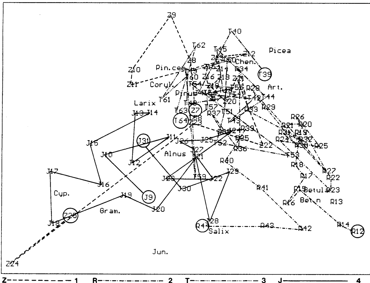
Fig. 11. Correspondence analysis. 1 - Roztoki a, 2 - Roztoki b, 3 - Tarnowiec, 4 - Jaslo
