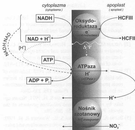
Rys. 1. Model aktywnego transportu azotanów do komórek roślinnych.
